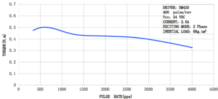
17HS5425 Torque Curve
